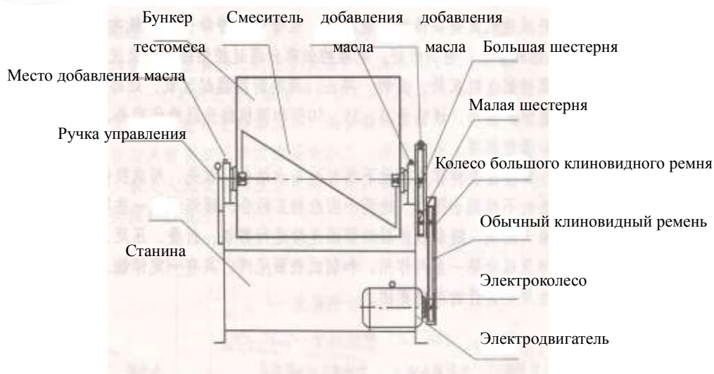
Схема конструкции машины HWY25
